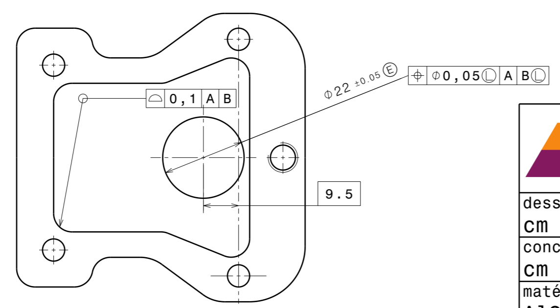
Vue de face.2 Echelle : 1:1
