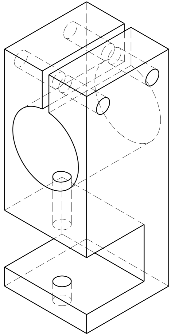
Vue isométrique Echelle : 1:1
