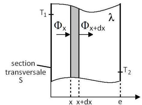
Figure 16. Conduction unidimensionnelle à travers une paroi plane
