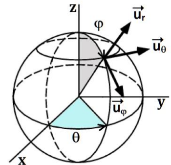
Figure 20. Repère sphérique
